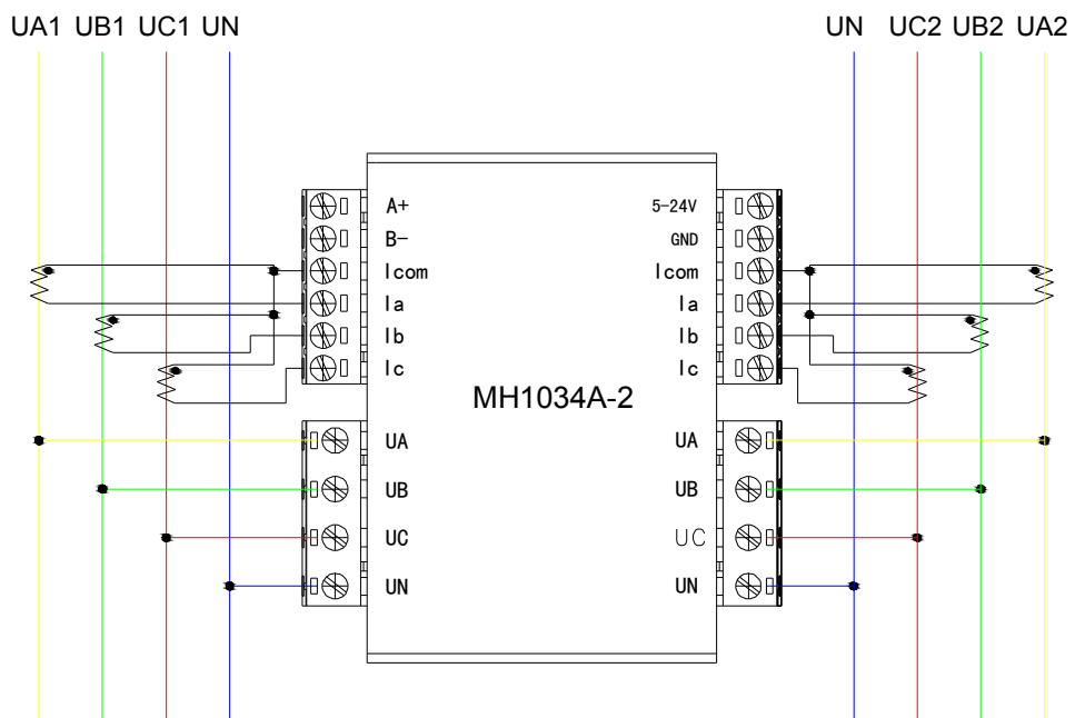
钳型互感器外接图
